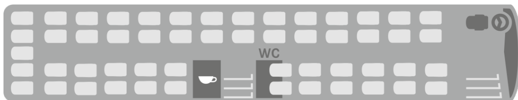
Variante 1: S 516 HD/2 - 3 Sterne - 53 Sitze + WC + Küche
