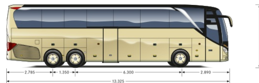
Alle Maße in Millimeter.
